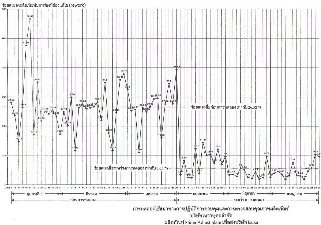
ภาพภาคผนวกที่ ก.1 กราฟแสดงร้อยละของผลิตภัณฑ์บกพร่องก่อนและระหว่างการทดลอง
