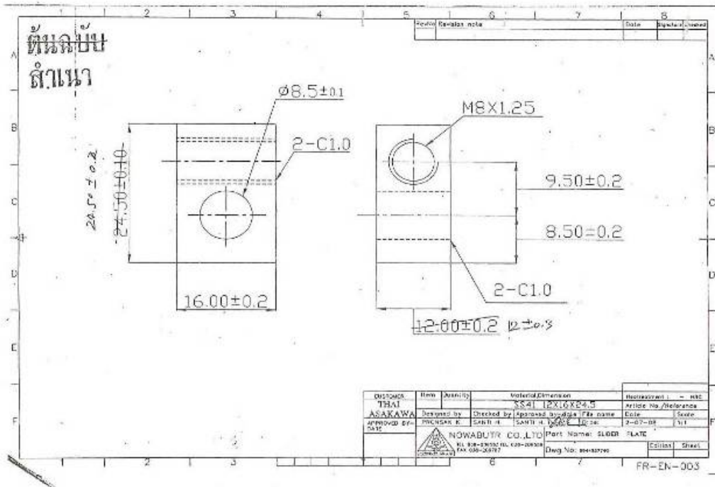
ภาพภาคผนวกที่ ก.2 แสดงแบบผลิตภัณฑ์ Slider Adjust Plate
